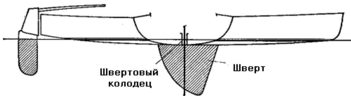
Рис. 5. Швертбот
