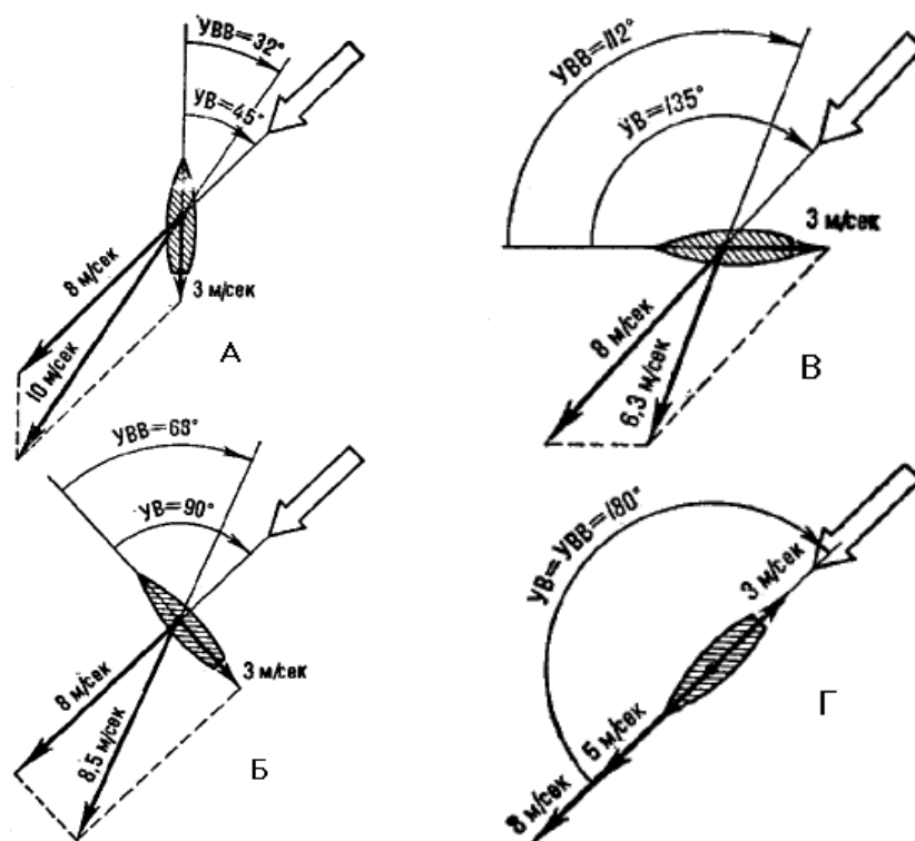
Рис. 90. Вымпельный ветер на разных курсах
