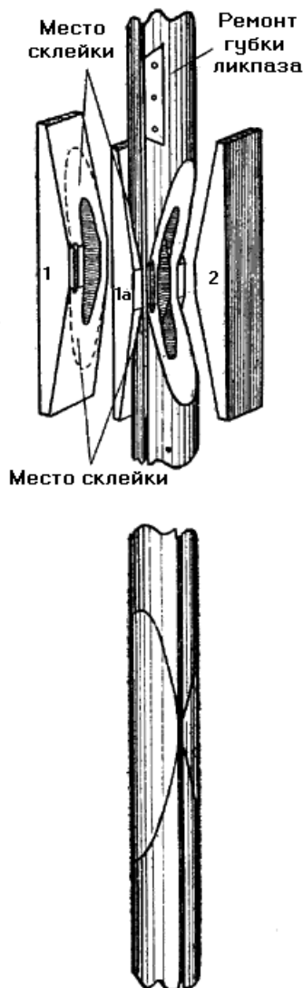
Рис. 74. Склеивание сломанной мачты
