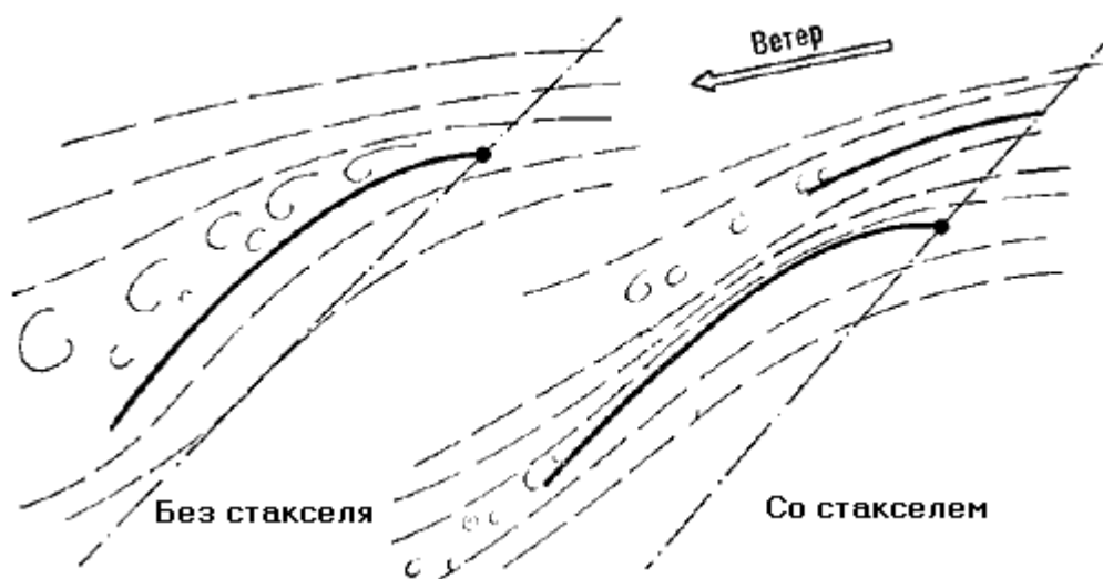
Рис. 97. Работа стакселя
