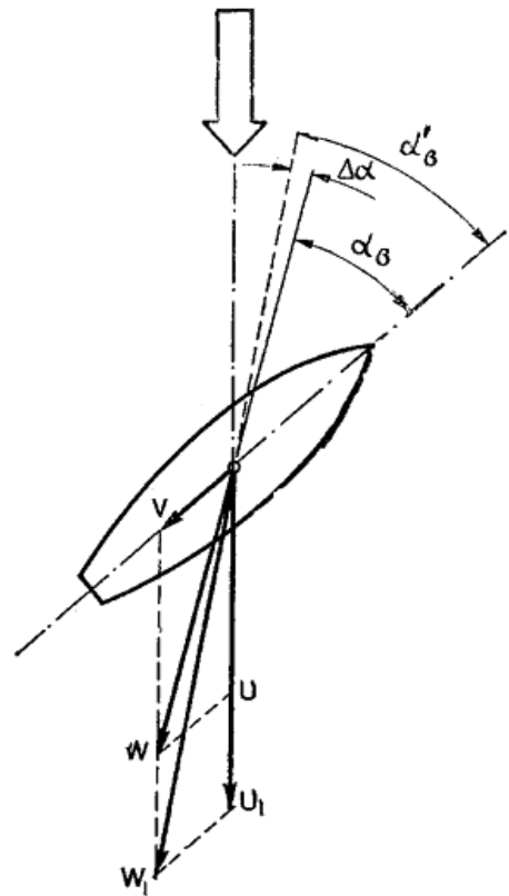
Рис. 92. В полосе сильного ветра можно идти круче
