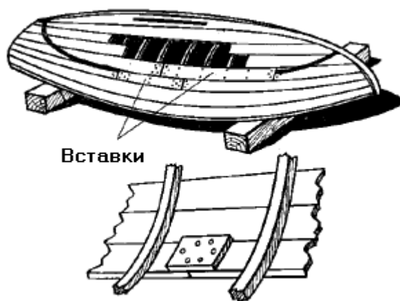
Рис. 73. Вставка в борту и способ
