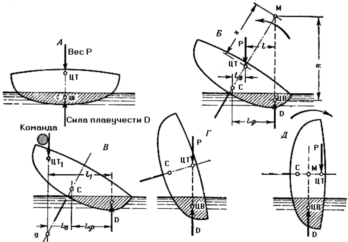
Рис. 78. Остойчивость швертбота
