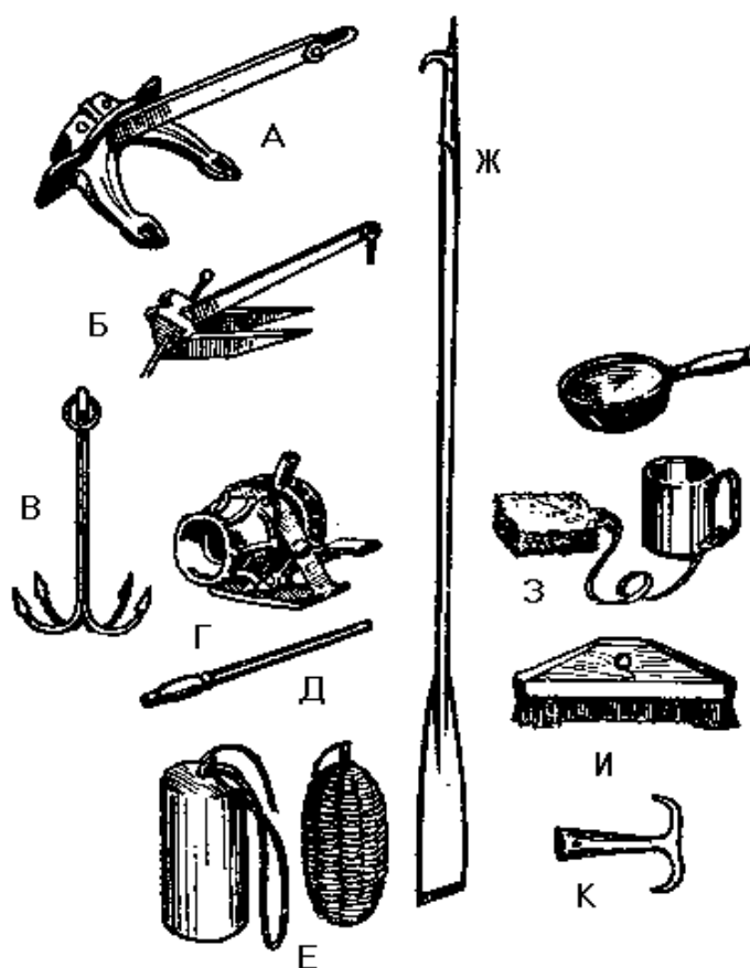
Рис. 54. Некоторые предметы снабжения и оборудования яхты:
