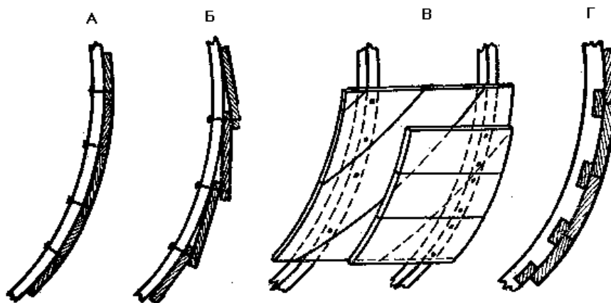
Рис. 29. Виды обшивки:
