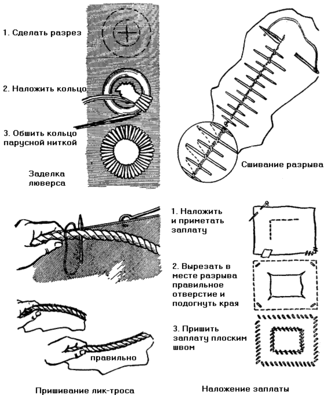
Рис. 72. Ремонт парусов
