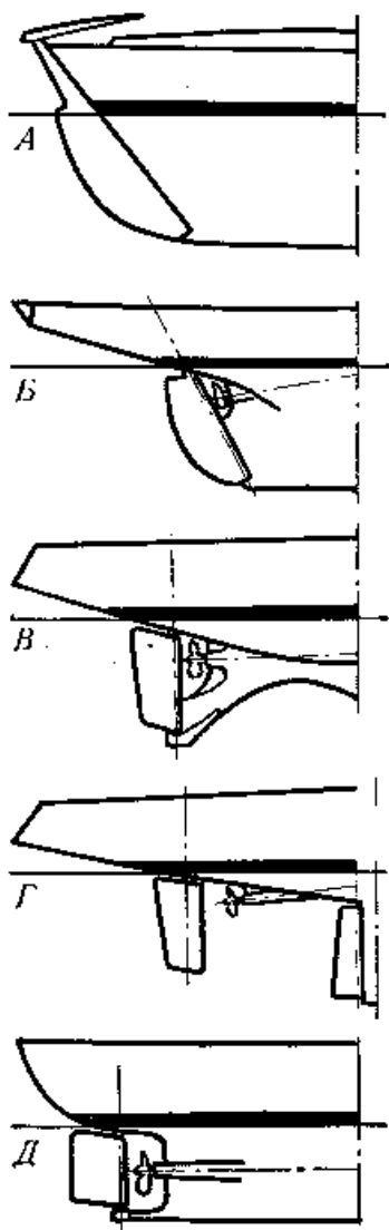
Рис. 30. Основные типы постоянных рулей:
