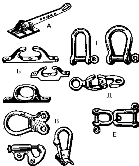
Рис. 51. Дельные вещи:
