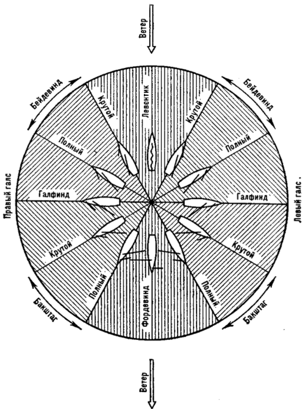
Рис. 101. Курсы и галсы яхты относительно ветра
