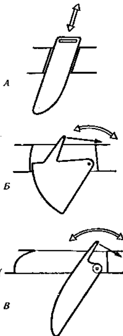
Рис. 33. Типы швертов: A — кинжальный; Б — качающийся секторный, В — качающийся мечевидный
