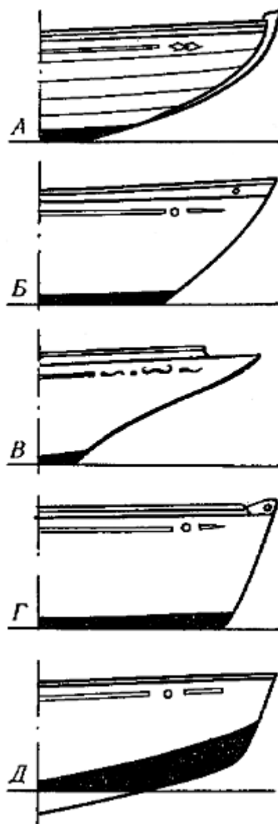
Рис. 11. Формы носовых частей: А — ложкаобразный штевень; Б — современный наклонный штевень; В — клипер-штевень; Г — прямой штевень; Д — транце вый нос (форшпигель) швертбота «Кадет»
