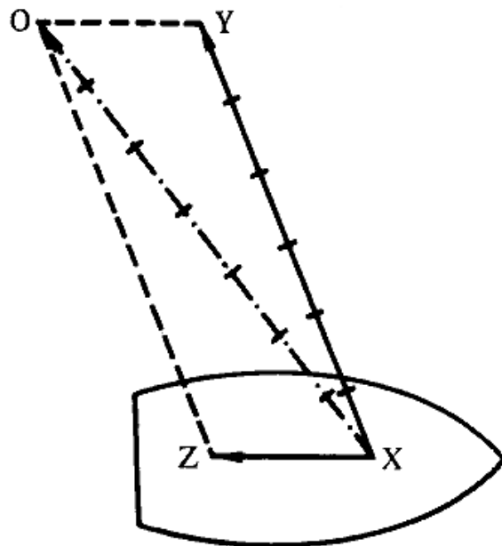
Рис. 15. Окончательная диаграмма вымпельного ветра.
