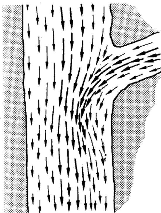
Рис 6. Влияние притока на течение реки.
