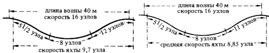
Рис. 29. Участок волны, на котором яхта может глиссировать или «сидеть» на волне.
