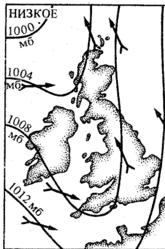
Рис. 65. V-образная депрессия, идущая над Исландией.
