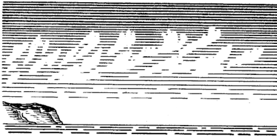
Рис. 61. Перистые облака, имеющие форму конских хвостов.
