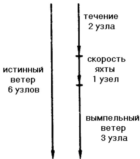
Рис. 16. Суммарное влияние течения и движения яхты на истинном ветре поперек течения и курса яхты. вымпельный ветер.
