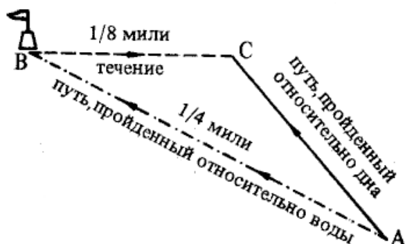
Рис. 20. Курс, пройденный относительно дна при учете течения.
