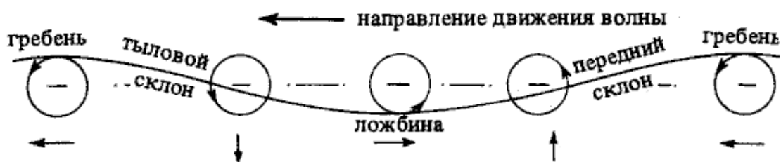
Рис. 35. Орбитальное движение частиц в волне. Основное направление движения на различных участках волны показано внизу стрелками.
